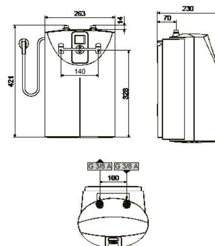
SNE 5 Dimensions
